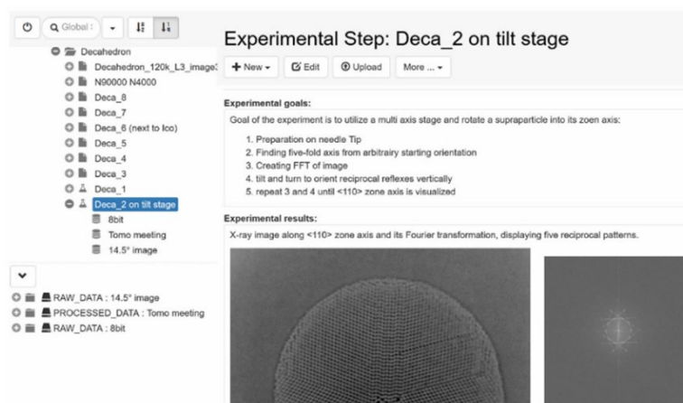
Abbildung 1: Benutzeroberfläche von openBIS aus der Perspektive der Forschenden. Im oberen linken Bereich ist die hierarchische Ordnerstruktur (Projekte, Experimente, Datensätze) dargestellt. Auf der rechten Seite werden strukturierte Metadaten (z.B. Probenparameter, Messbedingungen, Vorgehensweise) erfasst und mit den zugehörigen Daten verknüpft. Im gezeigten Beispiel handelt es sich um Röntgenmikroskopie-Daten, die als TIFF-Dateien vorliegen; sowohl die Rohdaten als auch die prozessierten Datensätze sind im System hinterlegt und werden im unteren linken Bereich visualisiert, sodass eine direkte Gegenüberstellung und Nachvollziehbarkeit der Verarbeitungsschritte möglich ist. Abbildung reproduziert aus [1].
